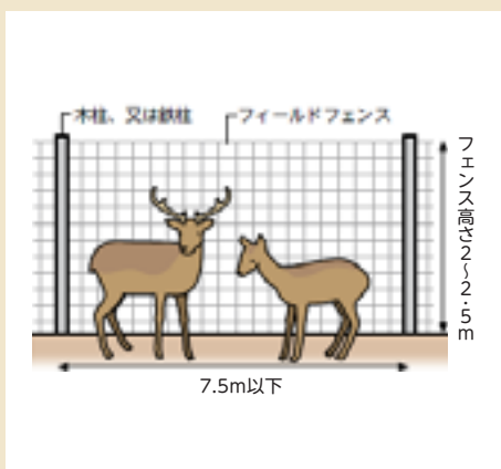
シカの金属柵設置イメージ
